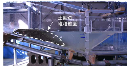
Fig.4 実験終了後の土砂の堆積状況 上: Case1-2, 下: Case5-2 Sediment deposition condition
